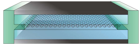
図1 端欠損を含むグラフェンナノリボンFET
