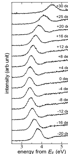
図 1 グラファイト 鏡像準位スペクトル
