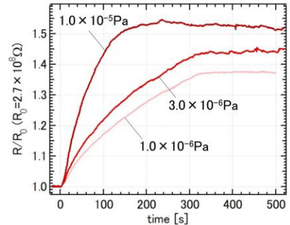
図2 90Kにて水曝露時の抵抗変化.
