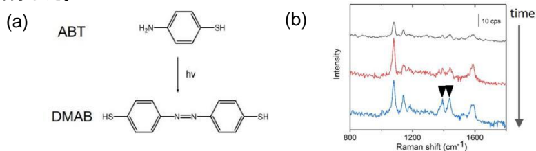
図 (a) ABT の光二量化反応。(b) ABT の SERS スペクトルの時間変化。DMAB 由来のピーク ( 1388\text{ cm}^{-1} 、 1438\text{ cm}^{-1} ) が時間の経過とともに増大した。
