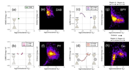
図 1. 電気伝導度 ( \log \sigma ) に対する分子軌道エネルギー ( \varepsilon ) の変化 (a, e) 1,4-dianobutane, (b, f) pyrazine, (c, g) 4,4' -bipyridine, (d, h) C 60
